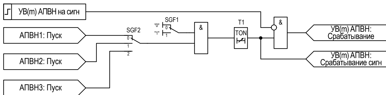
Рисунок 2.20 – Функциональная схема «УВ(м) АПВН»
