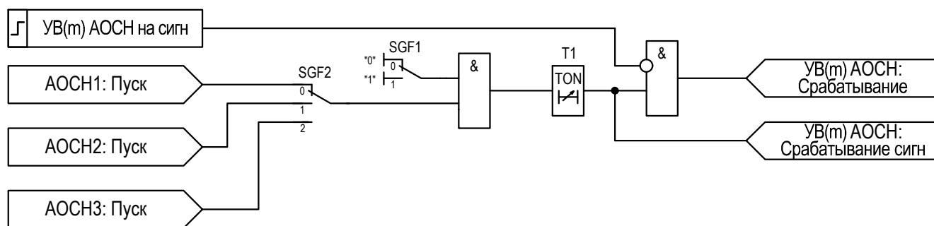
Рисунок 2.18 – Функциональная схема «УВ(м) АОСН»
