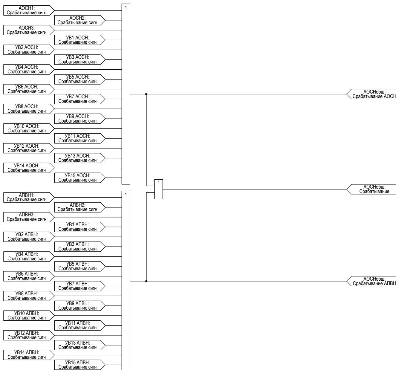
Рисунок 2.21 – Функциональная схема сборки сигналов АОСН
