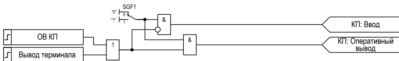
Рисунок 2.22 – Функциональная схема управления режимами работы «КП»
